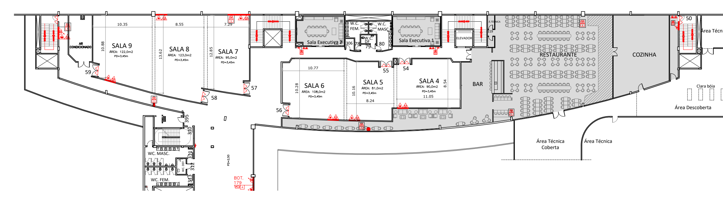
MEZANINO 1 ESCALA 1:400
