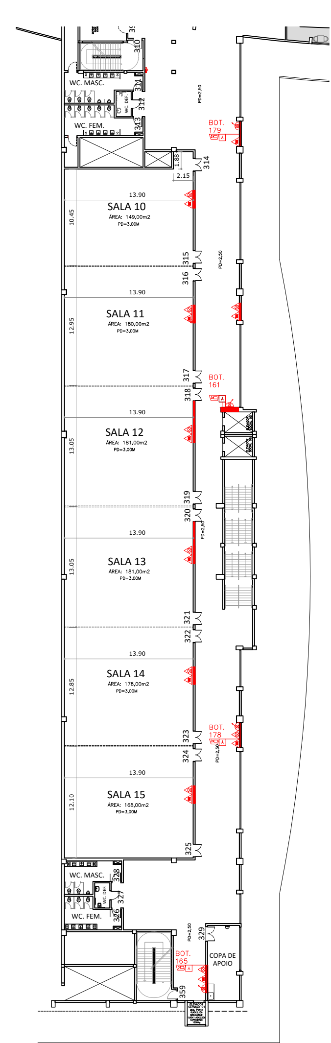
MEZANINO 2 ESCALA 1:400
