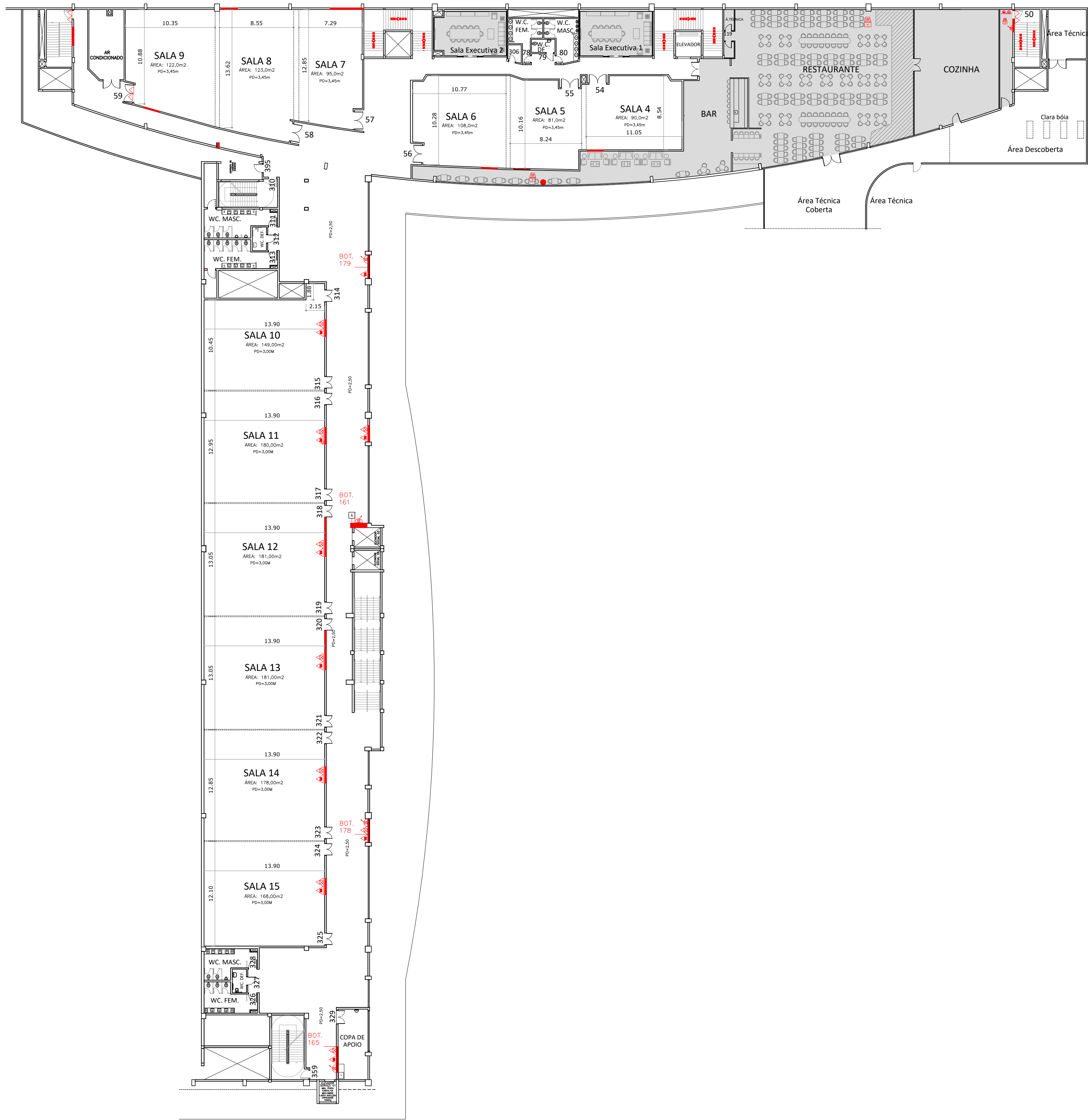
MEZANINO ESCALA 1:300
